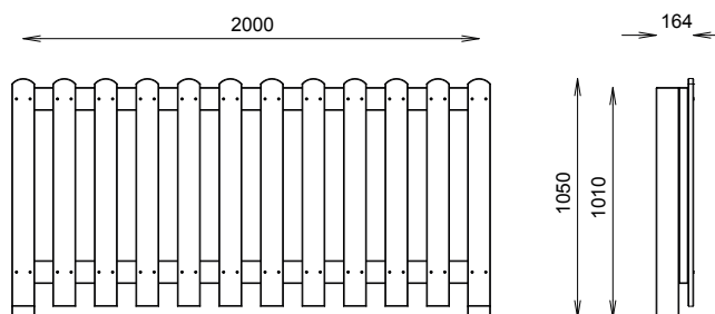
Schéma Clôture Ht. 100cm
